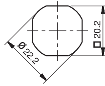
Geçiş ölçüsü
