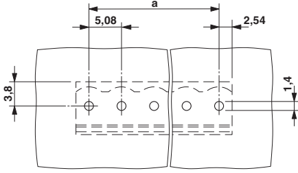
Delik şeması
