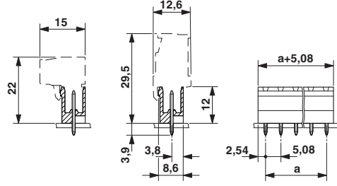
Boyutlu çizim
