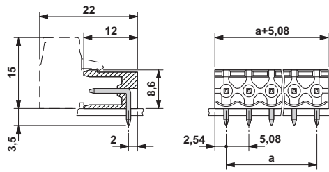
Boyutlu çizim
