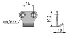
Karşılık sacı
