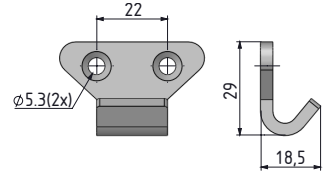
Karşılık sacı
