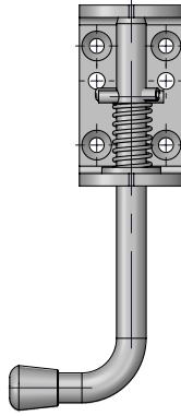
Açık pozisyon
