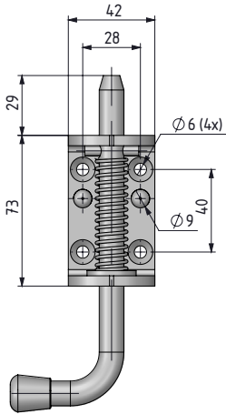
Kilitli pozisyon
