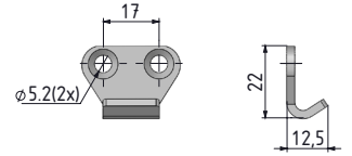
Karşılık sacı
