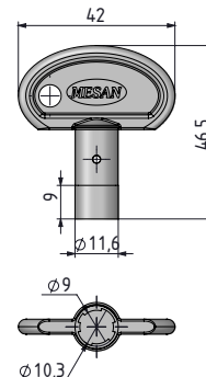
Tüp Anahtar
