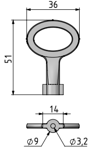
26713 3 mm Çentikli
