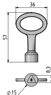
26738 8 mm Üçgen
