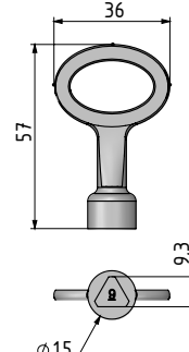
26739 9 mm Üçgen
