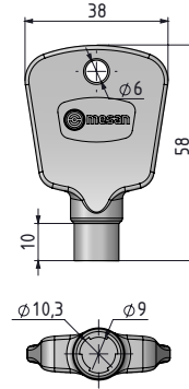
76993 Tüp Anahtar
