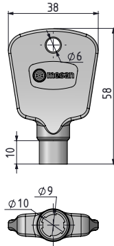
66993 Tüp Anahtar
