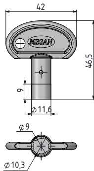
Tüp Anahtar
