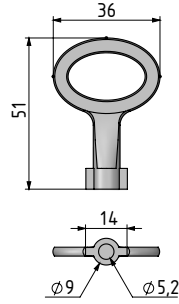
26715 5mm Çentikli
