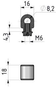
Çubuk tutucu
