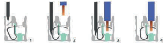
Yaylı Bağlantı
