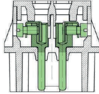
Vidalı Bağlantı
