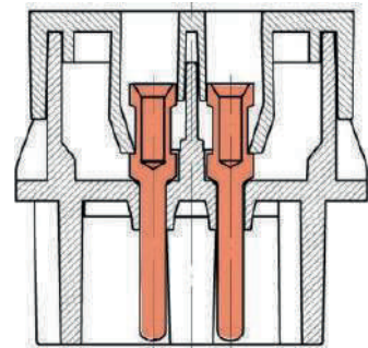
Krimp Bağlantı
