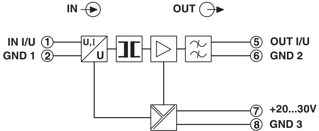
Devre diyagramı
