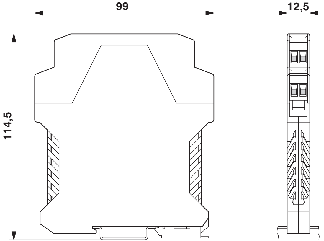
Boyutlu çizim
